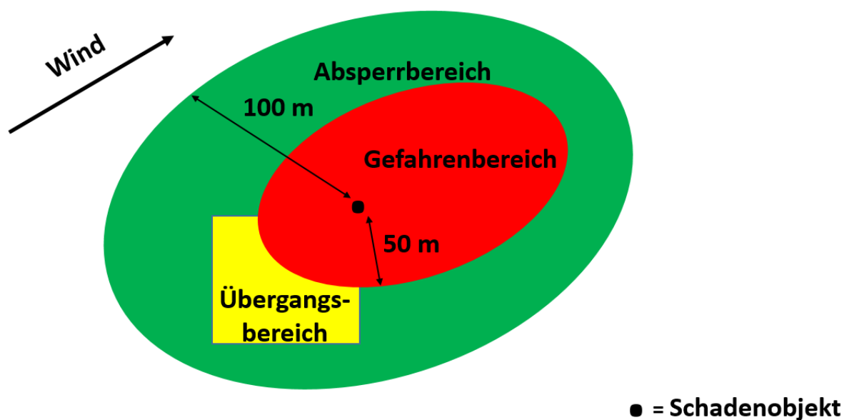
Abb. 10: Schematische Darstellung von Gefahren-, Übergangs- und Absperrbereich
